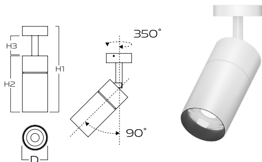
NLC-CAS24W - 4K H1 210 | H2 148 | H3 45 x D73mm
