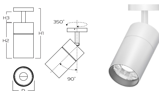
NLC-CAS36W - 4K H1 227 | H2 160 | H3 50 x D90mm
